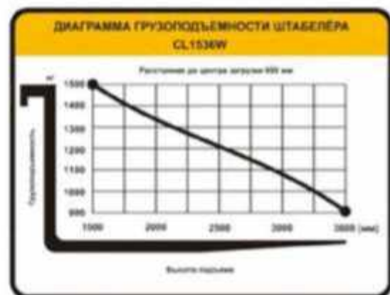
Рисунок 4. Основные параметры штабелера.
