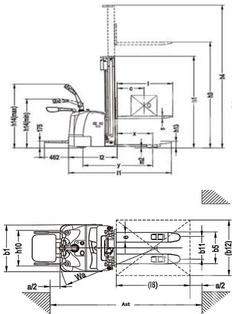
Рис. 1 Габаритные размеры штабелера
