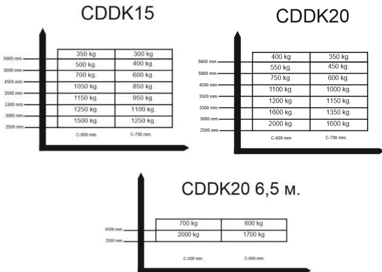
Рис. 2, 3, 4 – Кривые грузоподъемности
