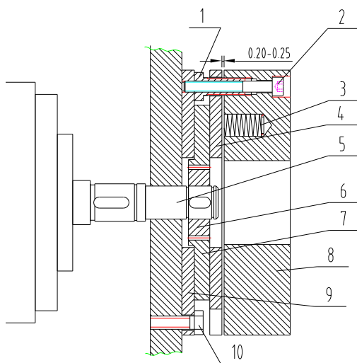
Рис.8 - Регулировка зазора в тормозном механизме
