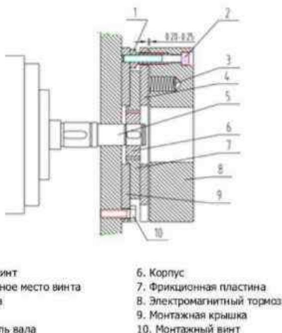
Рисунок 11. Регулировка зазора.
