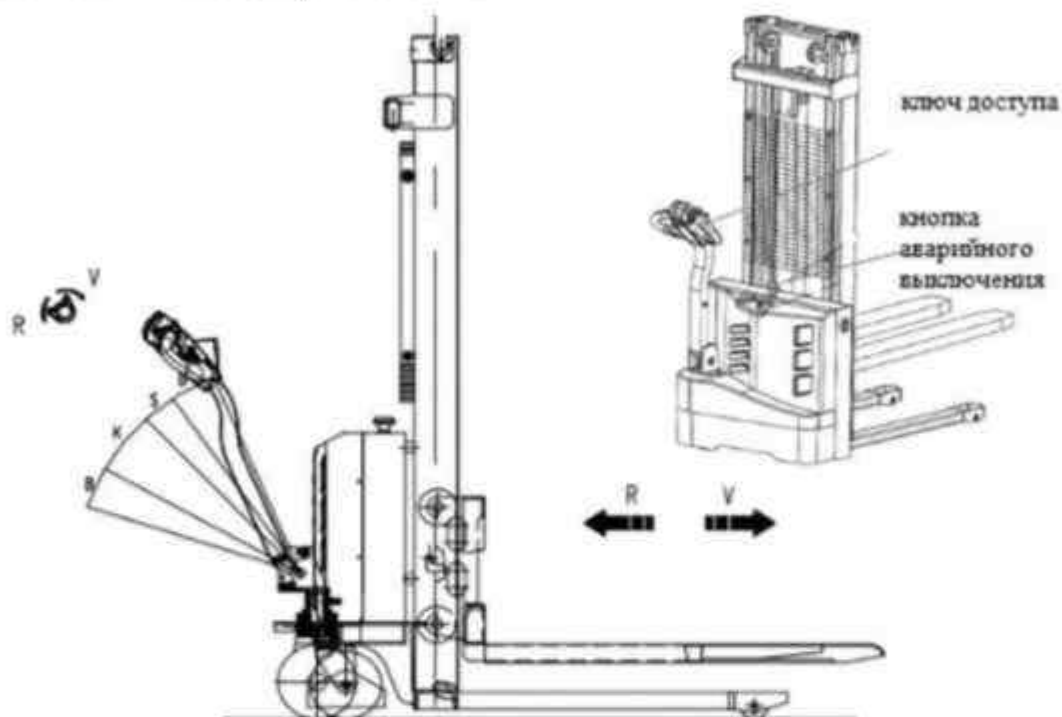
Рисунок 5. Органы управления.
