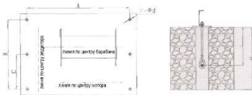
Рисунок 6. Разметка крепежных болтов.
