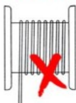
Рисунок 7. Правильность намотки грузоподъемного каната.
